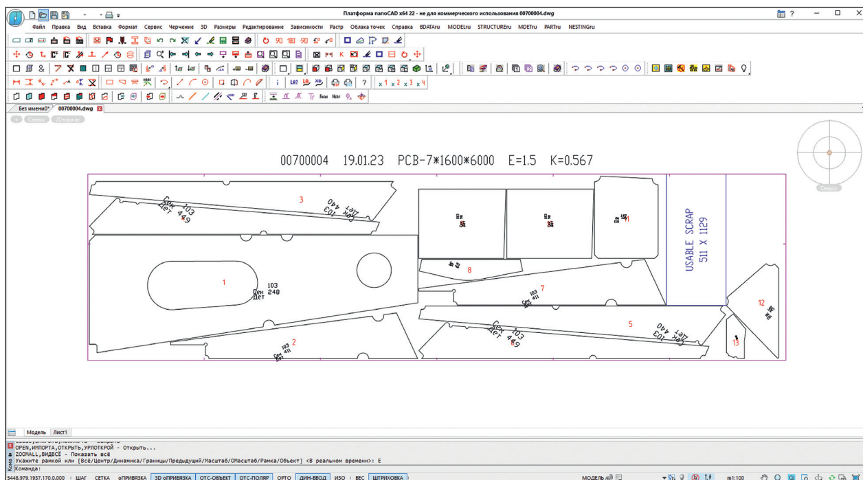
Рис. 1. Карта раскроя листового проката
